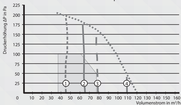
Volumenstromkennlinien Fox Comfort plus
