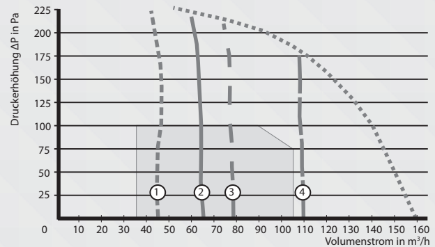
Volumenstromkennlinien Fox Comfort 150
